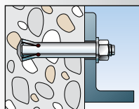
kotva zirkon FZA
